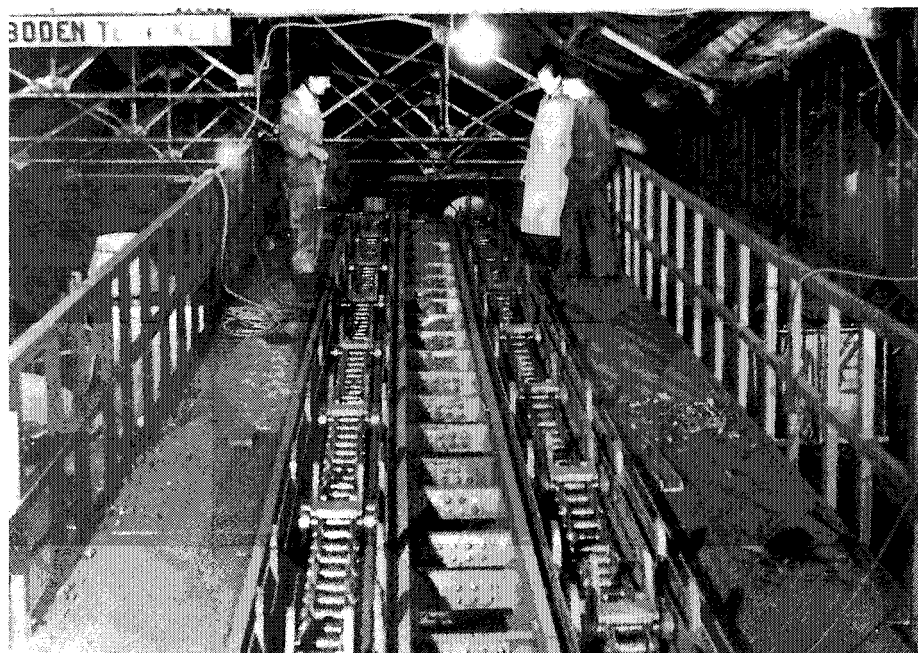
Afb. 75. kettingbaan
