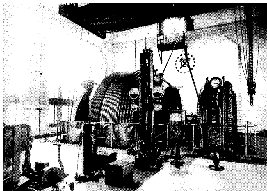
Afb. 70. ophaalmachine
