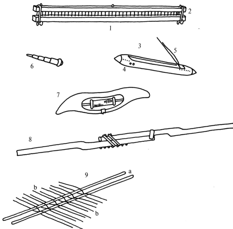
Afb. 62. effenaar, weefspoel, tempel en dradenkruis met kruisroede
