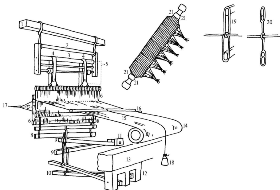
Afb. 58. weefkam
