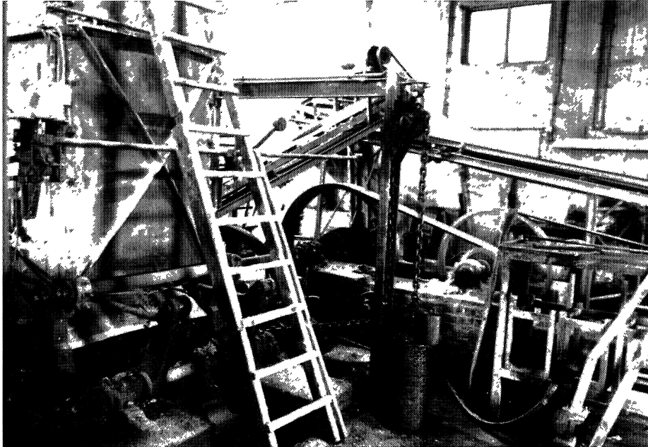
Afb. 22. Aberson-vormbakpers
