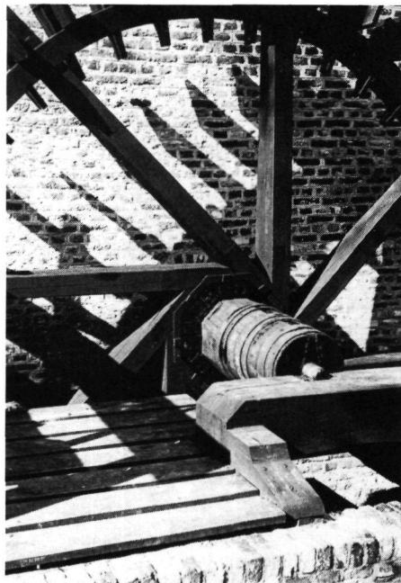
Afb. 73. naaf en spaken van het molenrad van de watermolen te Baarlo
