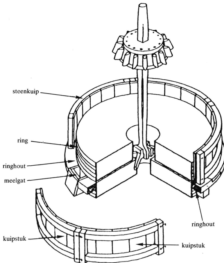
Afb. 81. steenkuij
