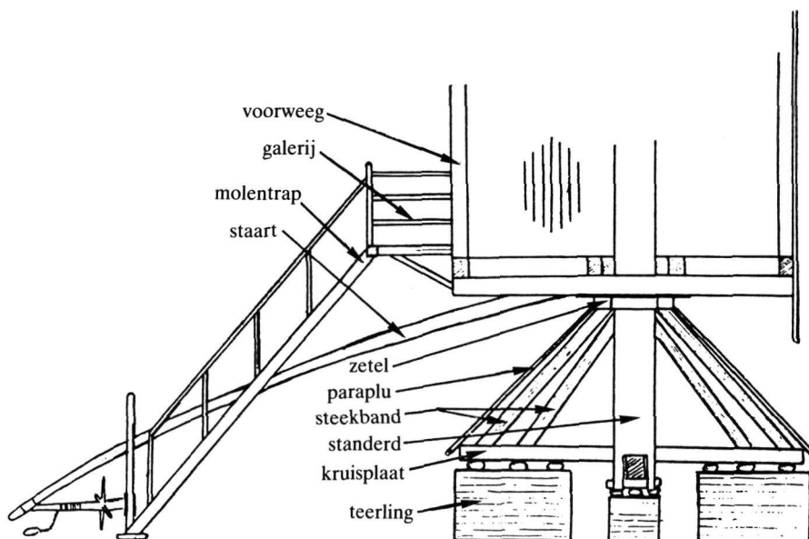
Afb. 22. stander en staart van de standermolen
