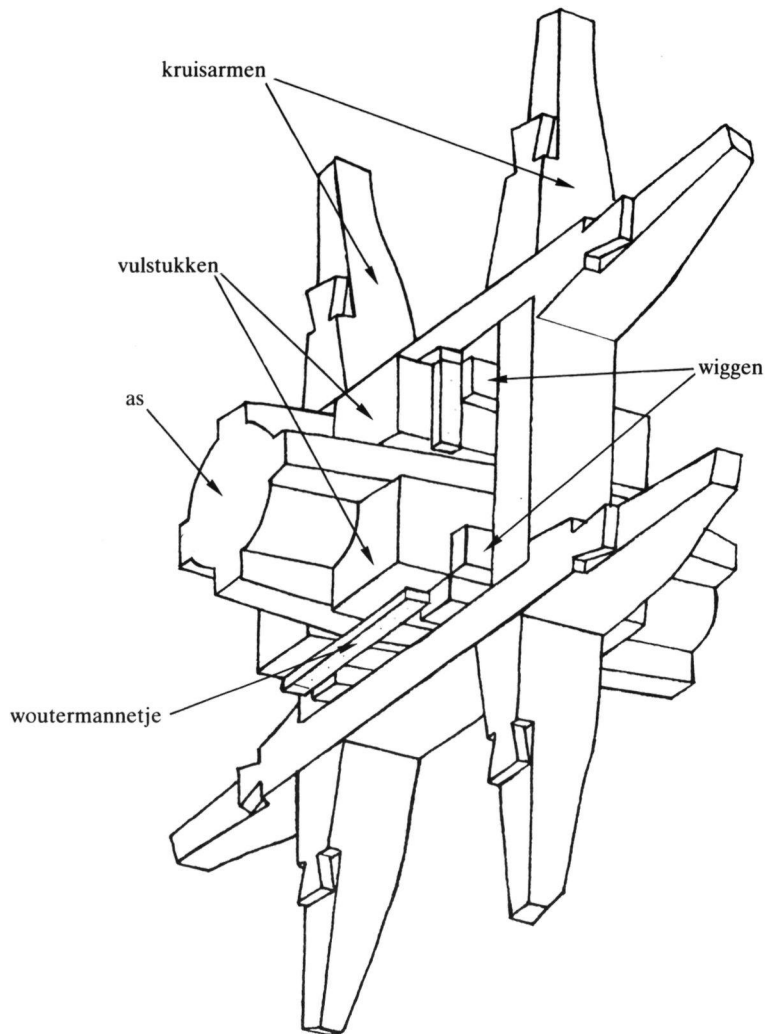
Afb. 50. bevestiging aswiel
