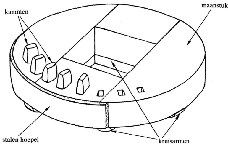
Afb. 60. bonkelaar
