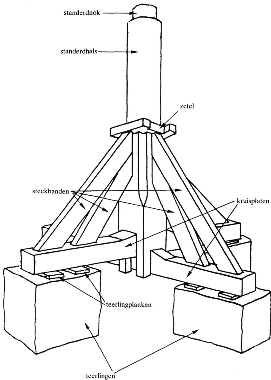
Afb. 12. standerd
