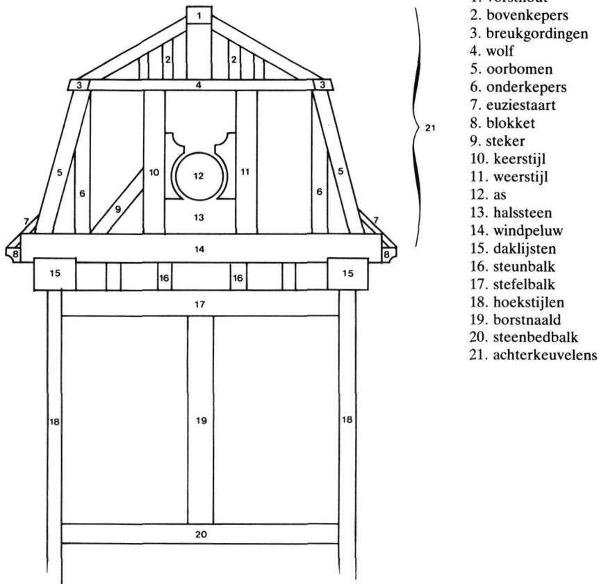
Afb. 18. stormeinde
