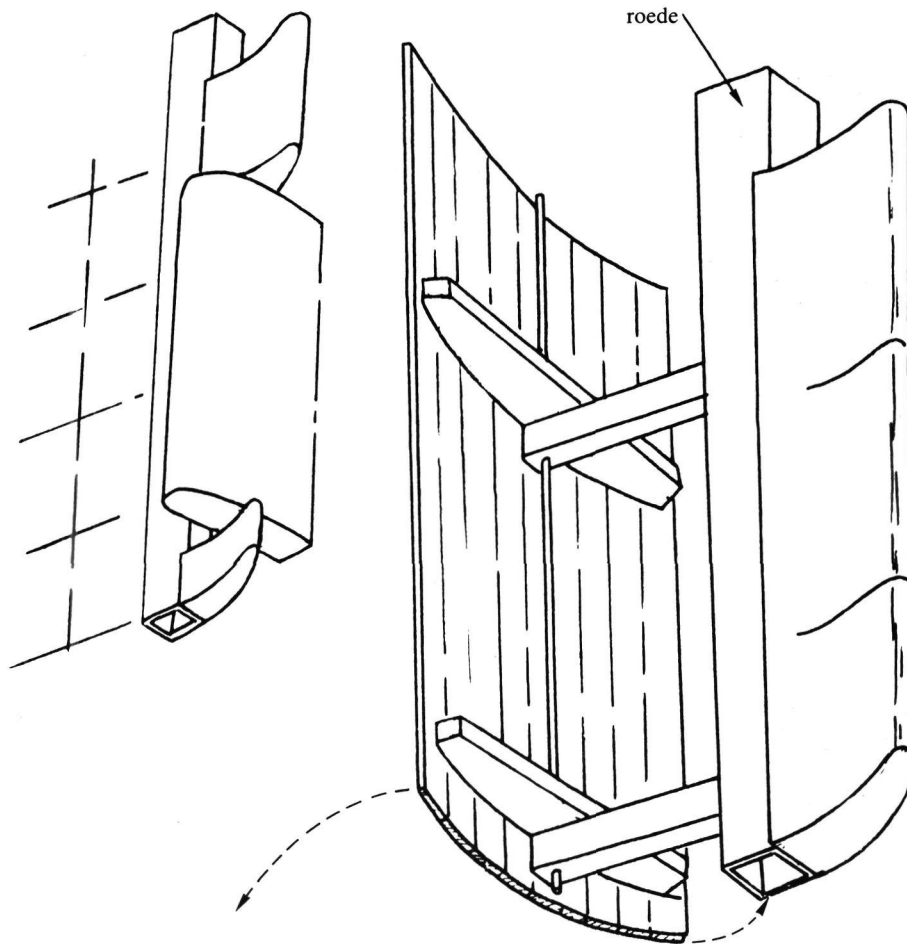
Afb. 41. kleine remklep (links) en geopende remklep (rechts) bij zelfzwichtingroede
